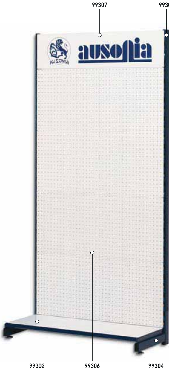
Espositore metallo versione standard (dim. LxHxP: cm 100x200x40) Metal display (WxHxD: cm 100x200x40) Composizione base: Basic components: Montante cm 196 (2 pz) 99301 Lateral frame cm 196 (2 pcs) Ripiano cm 97x40 (1 pz) 99302 Shelf cm 97x40 (1 pc) Mensola per base terra (2 pz) 99304 Basement shelf (2 pcs) Schienale forato cm 97x42 (4 pz) 99306 Back panel cm 97x42 (4 pcs) Schienale serigrafato (1 pz) 99307 Panel with logo (1 pc) Accessori: Accessories: Gancio singolo 99161 Simple hook Staffa per ripiano addizionale 99305 Stirrup for additional shelf
